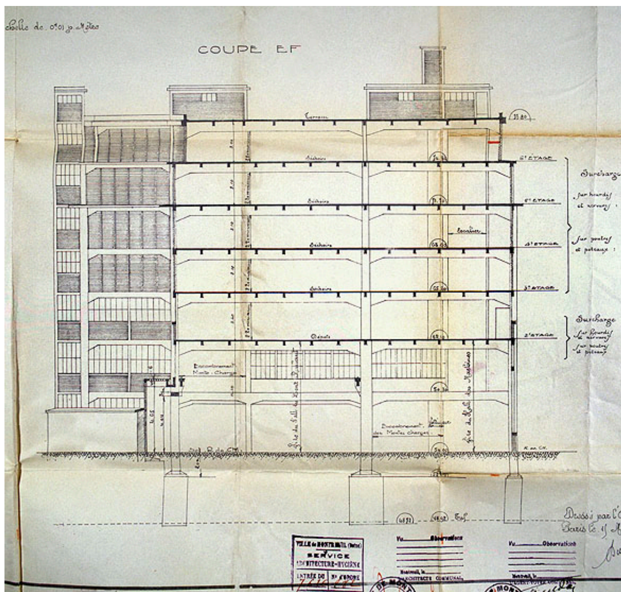
Coupe du bâtiment nord, 1927, archives municipales de Montreuil.
