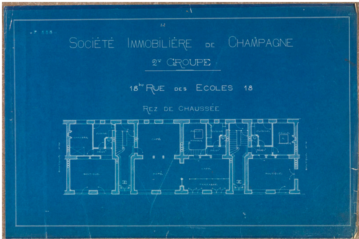
Plan. Société immobilière de Champagne. Rez-de-chaussée. 2e groupe, 18 rue des écoles.
