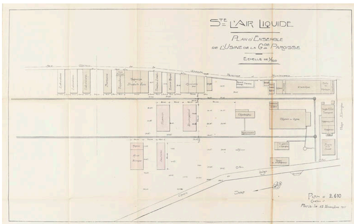
Plan d'ensemble de l'usine N°2.610.
