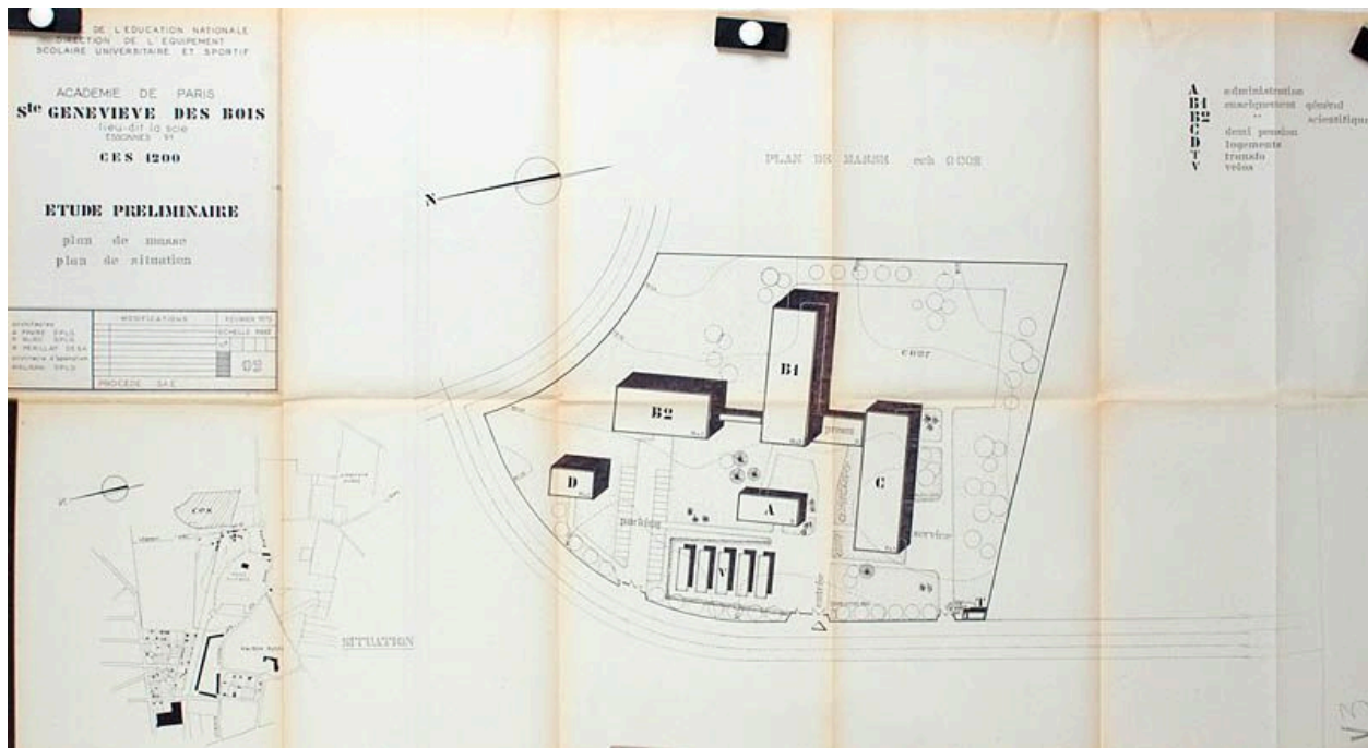
Plan masse et de situation du CES 1200, collège Paul Eluard.
