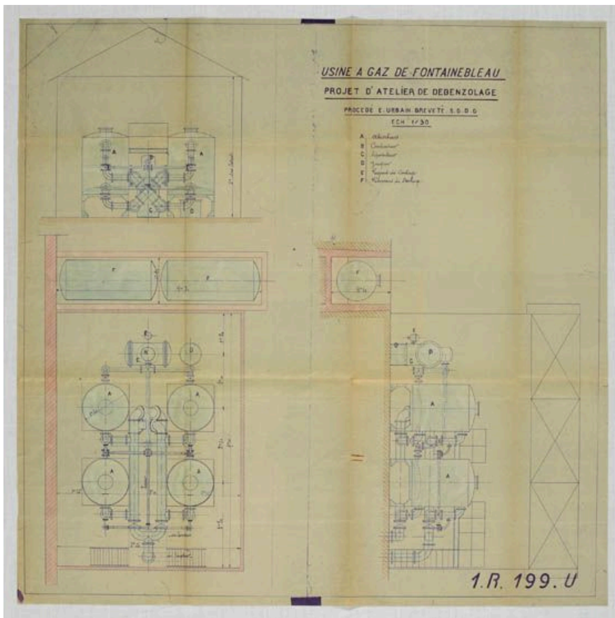
Plan et coupe de l'atelier de débenzolage de l'usine à gaz à Fontainebleau, 1928. (AD Seine-et-Marne, 5MP185)
