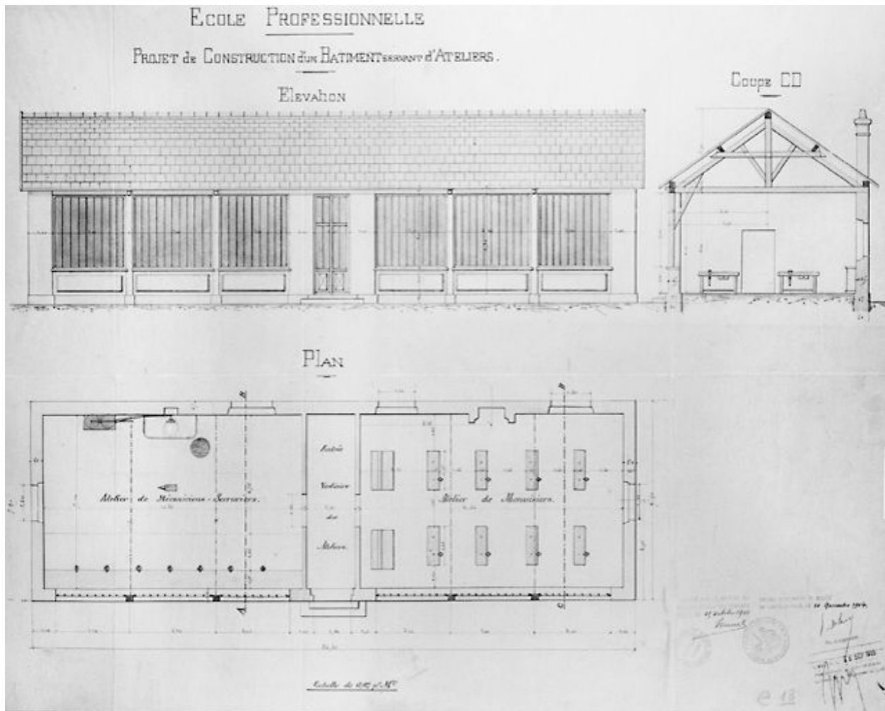
Collège de Melun. Ecole professionnelle. Projet de construction d'un bâtiment servant d'ateliers. Calque aquarellé, 15 octobre 1904. (AM Melun. 1 Fi 527)
