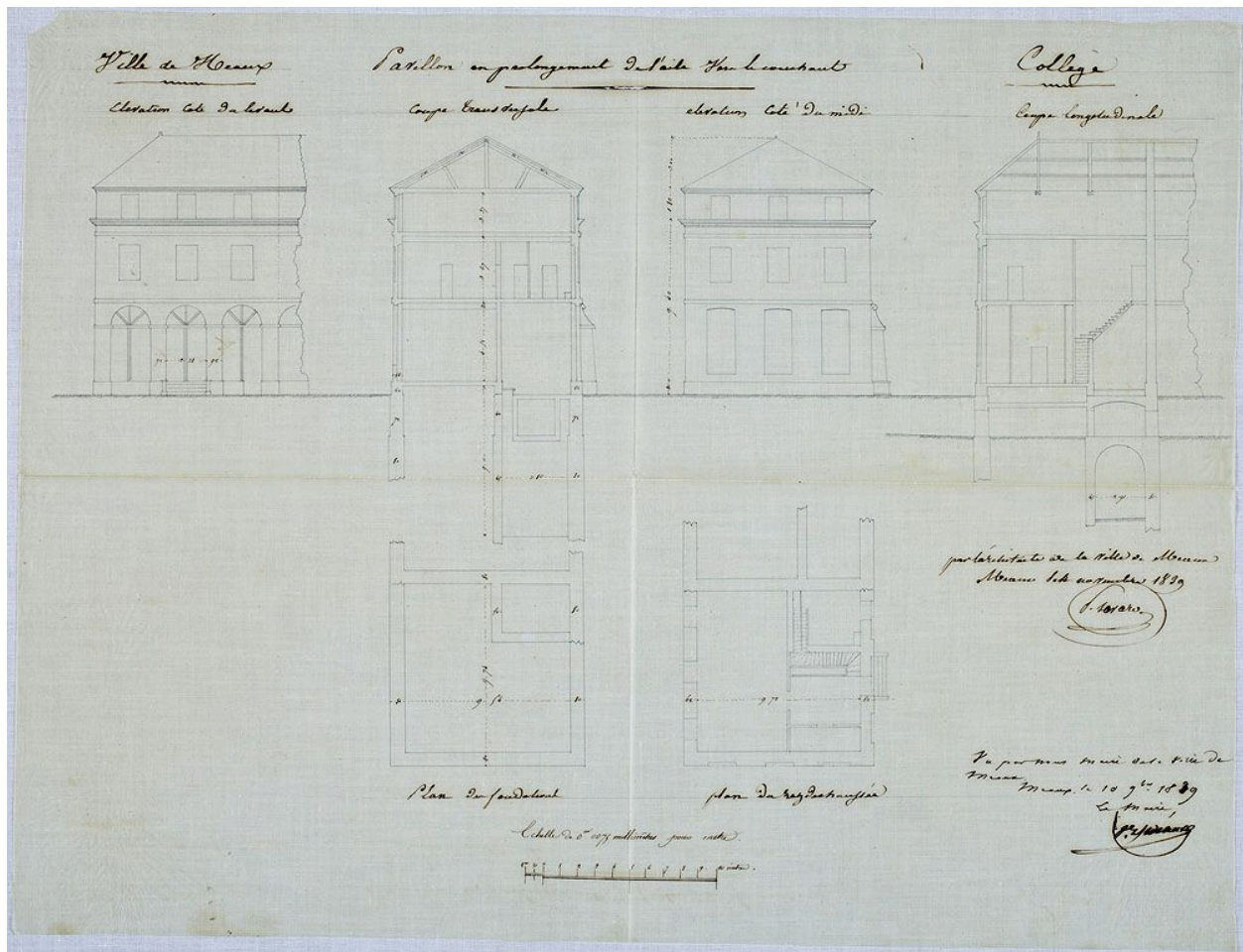
Collège, pavillon en prolongement de l'aile sur le couchant ( 2 élévations, 2 coupes, 2 plans). 1839. Papier aquarellé. (AD Seine-et-Marne. 4 Op 284/4)
