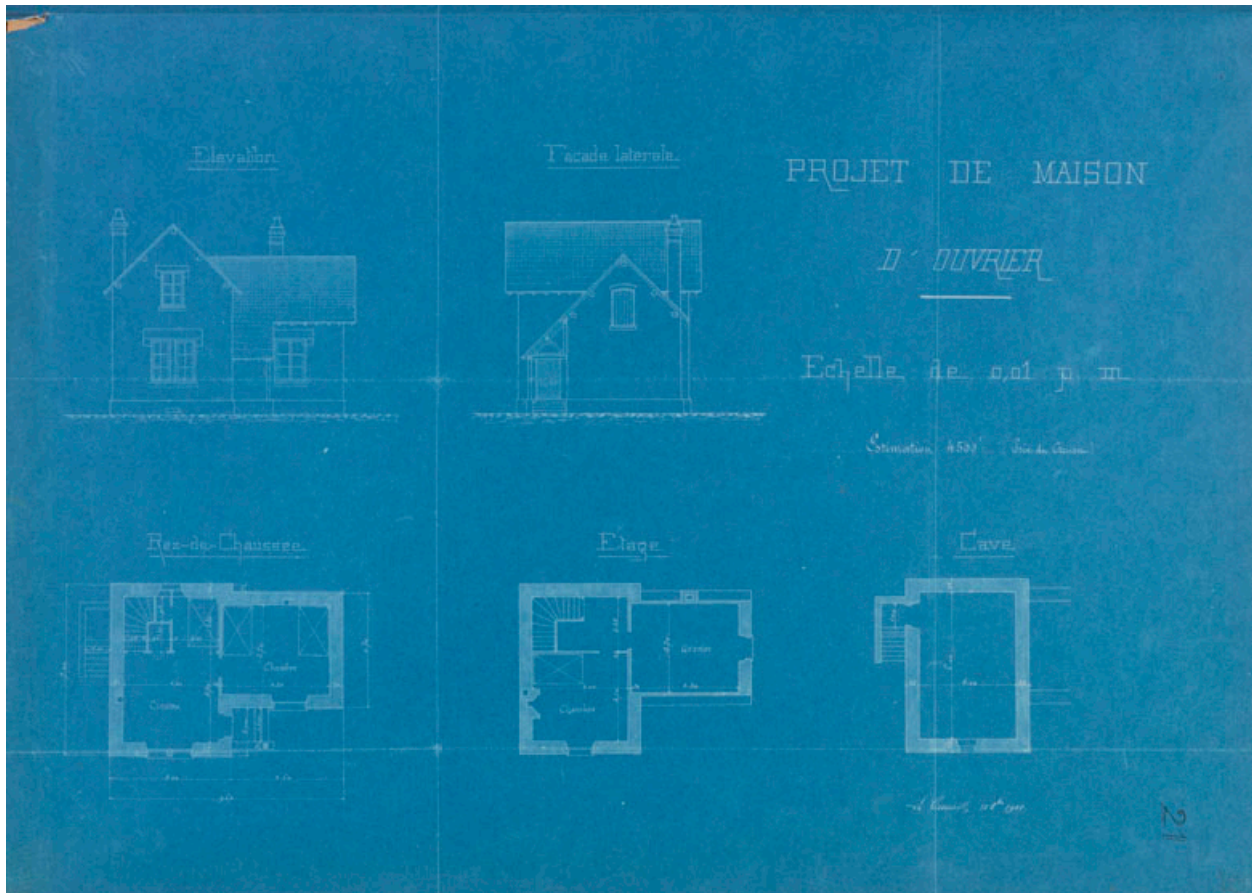
Plan. Edmond Delaire. Projet pour "le nouveau quartier" de Champagne-sur-Seine. Projet de maison d'ouvrier.
