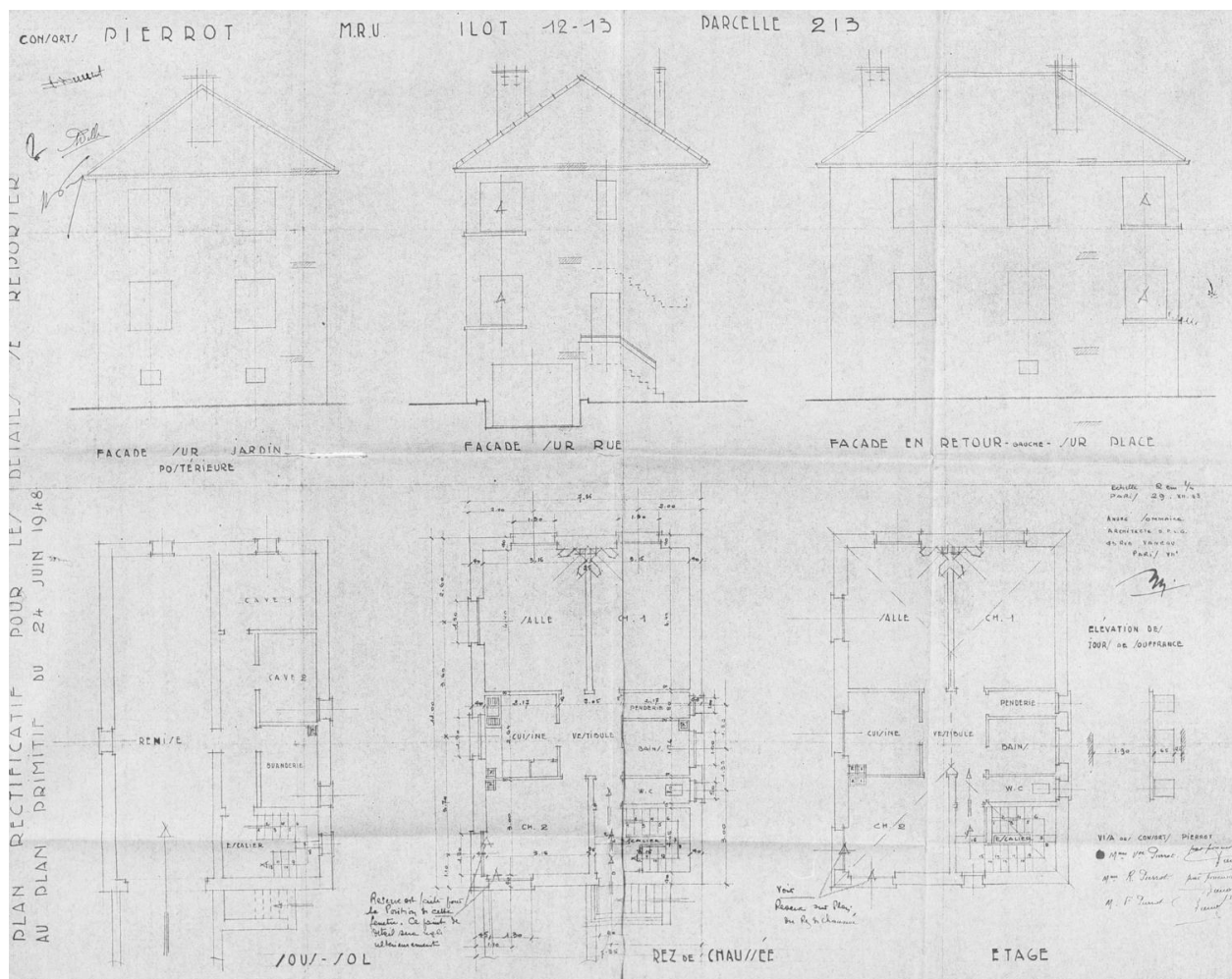
Elévations et plans de la maison reconstruite dans l'îlot 12, parcelle 215, pour les consorts Pierrot (9, rue Paul-Henri-Challine) ; L. Mendelssohn, architecte en chef, P. Garofalo, architecte chef de groupe, A. Sommaire, architecte d'opération ; plan modifiant le plan primitif du 24 juin 1948.
