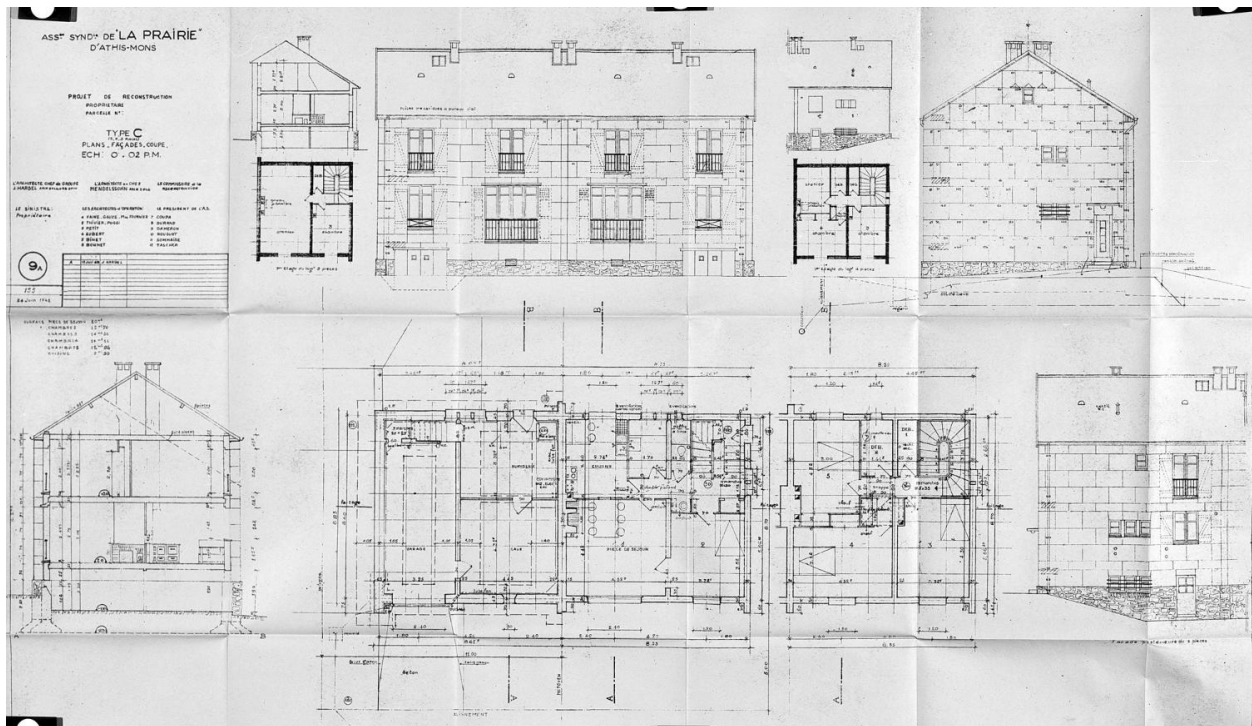
Pavillons de type C ; plans, façades et coupe ; 1948.
