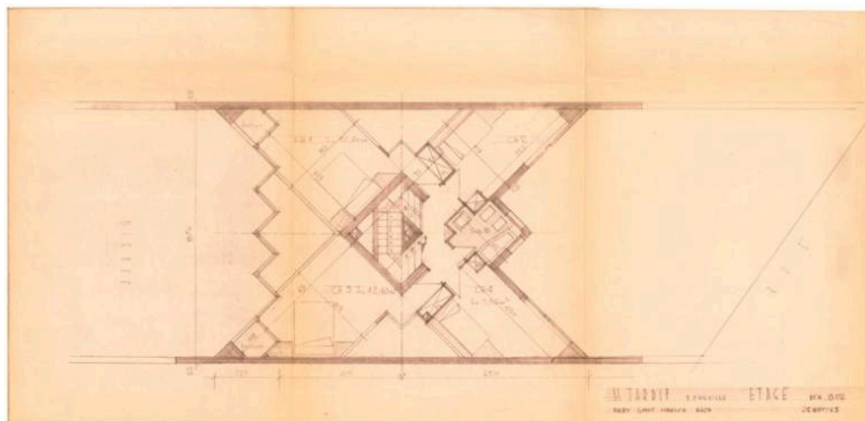
Plan de l'étage (extrait du permis de construire).
