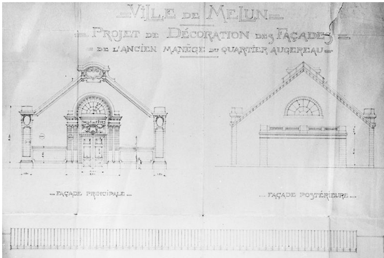
Projet de Daniel Beylard pour la transformation du manège de cavalerie en salle des fêtes (20 avril 1911) : la façade principale et la façade postérieure. (AM Melun. 1 Fi 895)
