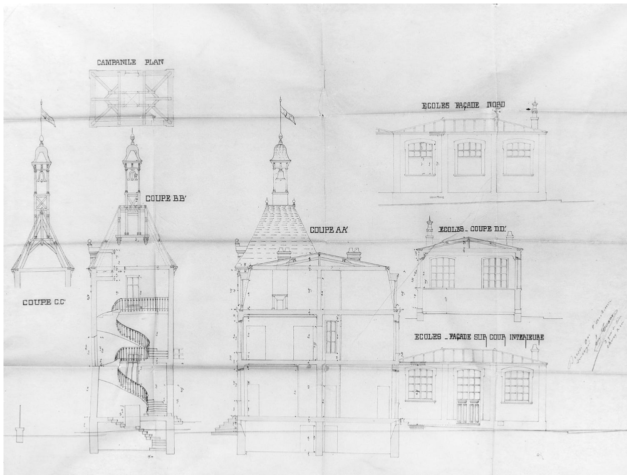
Projet de l'architecte Eugène Tuane : coupes et façades des écoles, 20 juin 1876.
