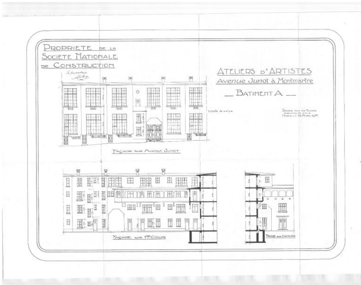
Relevé des façades du bâtiment A
