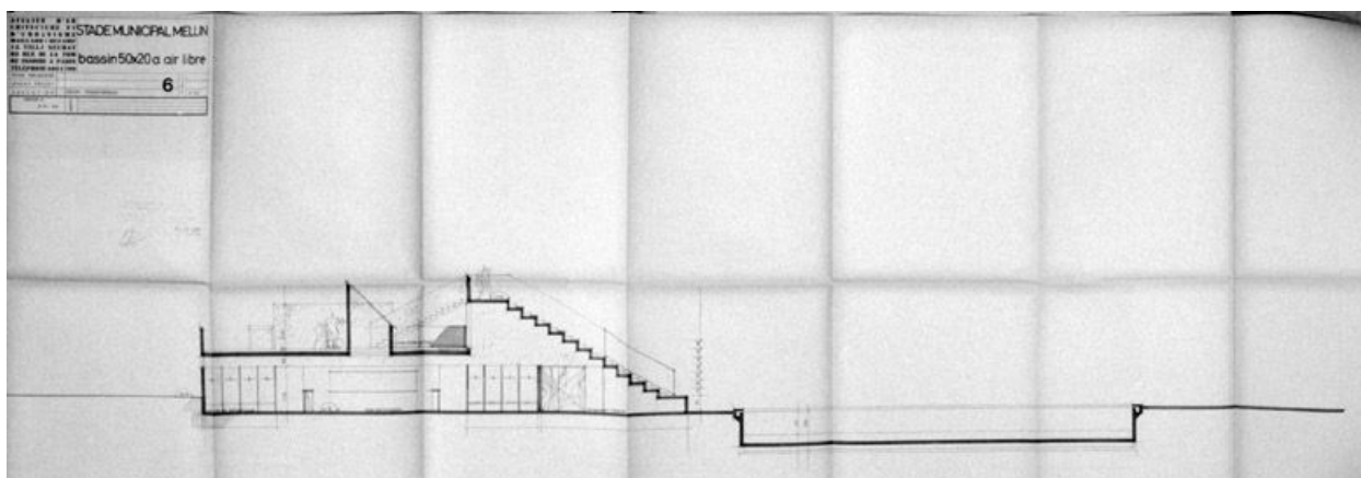
Bassin découvert : coupe. Tirage d'architecte, 14 octobre 1966. (AM Melun. 466 W 84)
