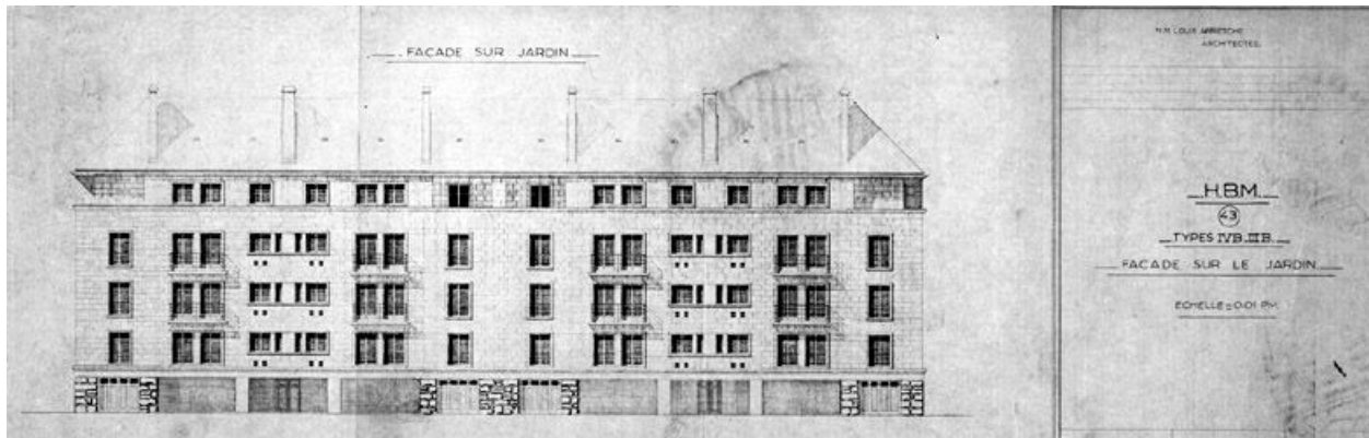
Projet de Louis Arretche pour un immeuble HBM, types III B et IV B : façade sur jardin. Tirage d'architecte, 1948. (AM Melun. 1 Fi 1311)
