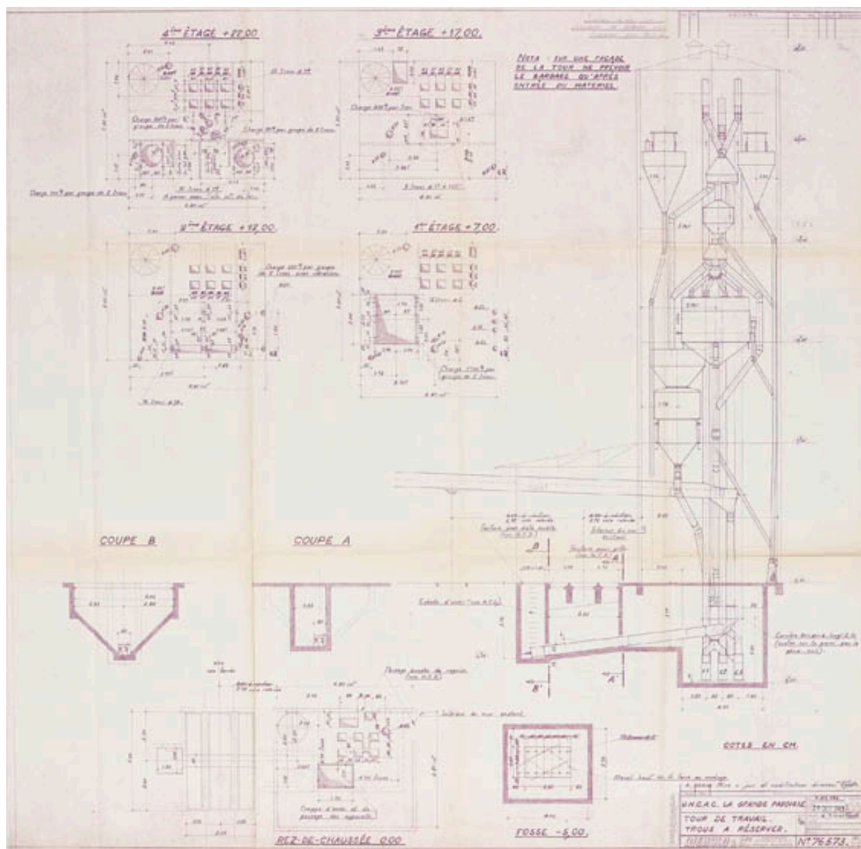
Silos de l'UNCAC de la Grande Paroisse. Tour de travail. Trous à réserver. Echelle 1/50e. 29 octobre 1963. (Archives départementales).
