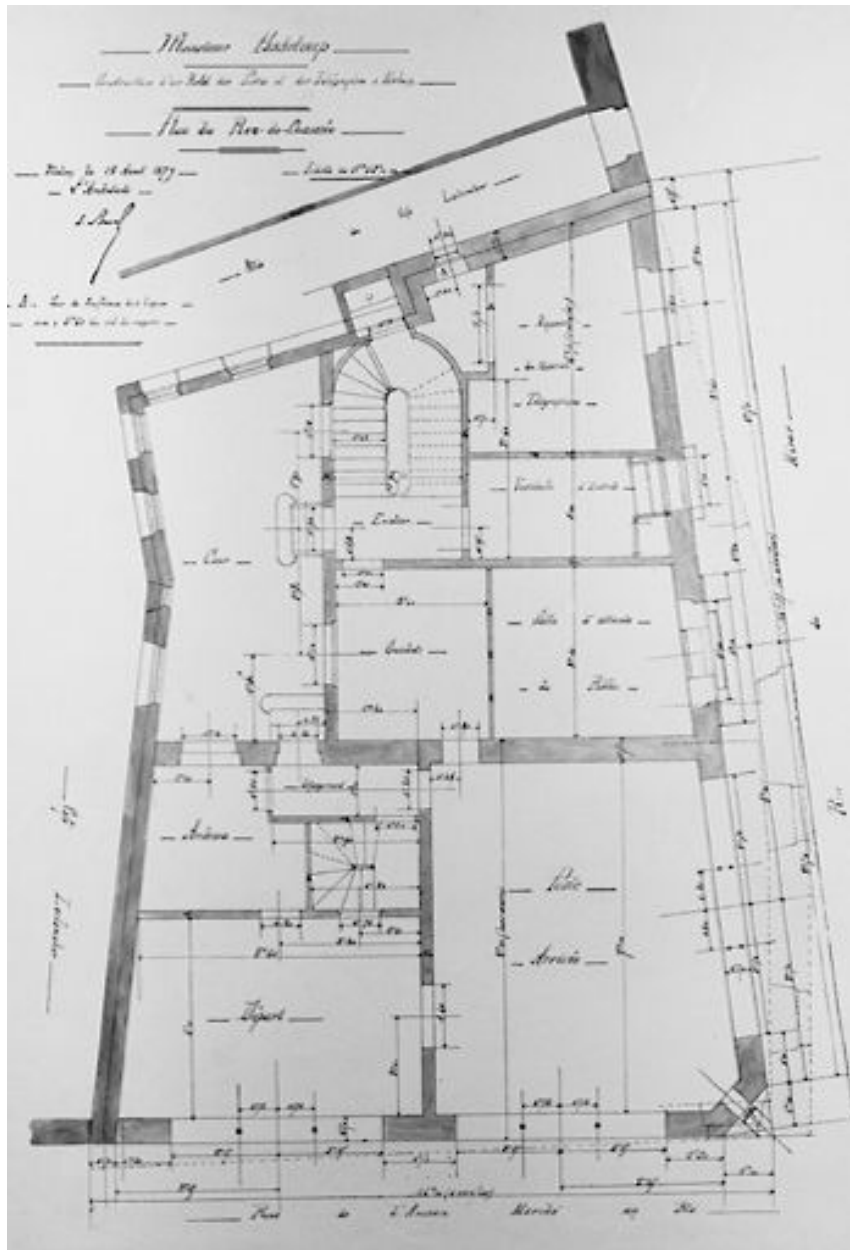
Monsieur Padeloup. Construction d'un hôtel des postes et télégraphes à Melun, rue de l'ancien marché au blé. Plan du rez-de-chaussée. Papier, 1879 (15 août). (AM Melun. 1 Fi 827)
