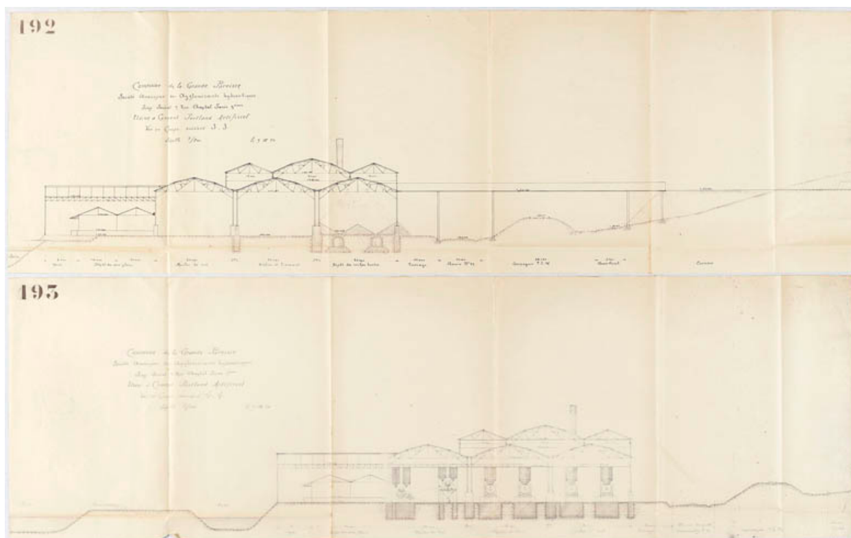
Cimenterie de la Grande Paroisse. Plans vues en coupe. échelle 1/200e. (archives départementales).
