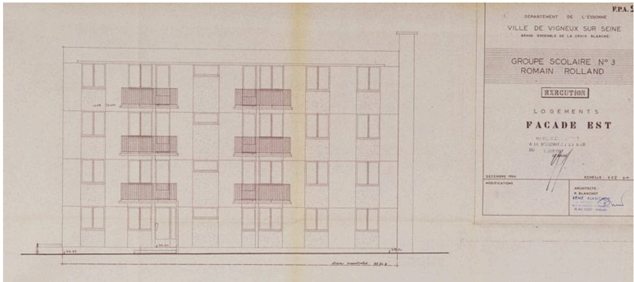
Plan de la façade est du bâtiment des logements. (AD Essonne, 1051 W 200)
