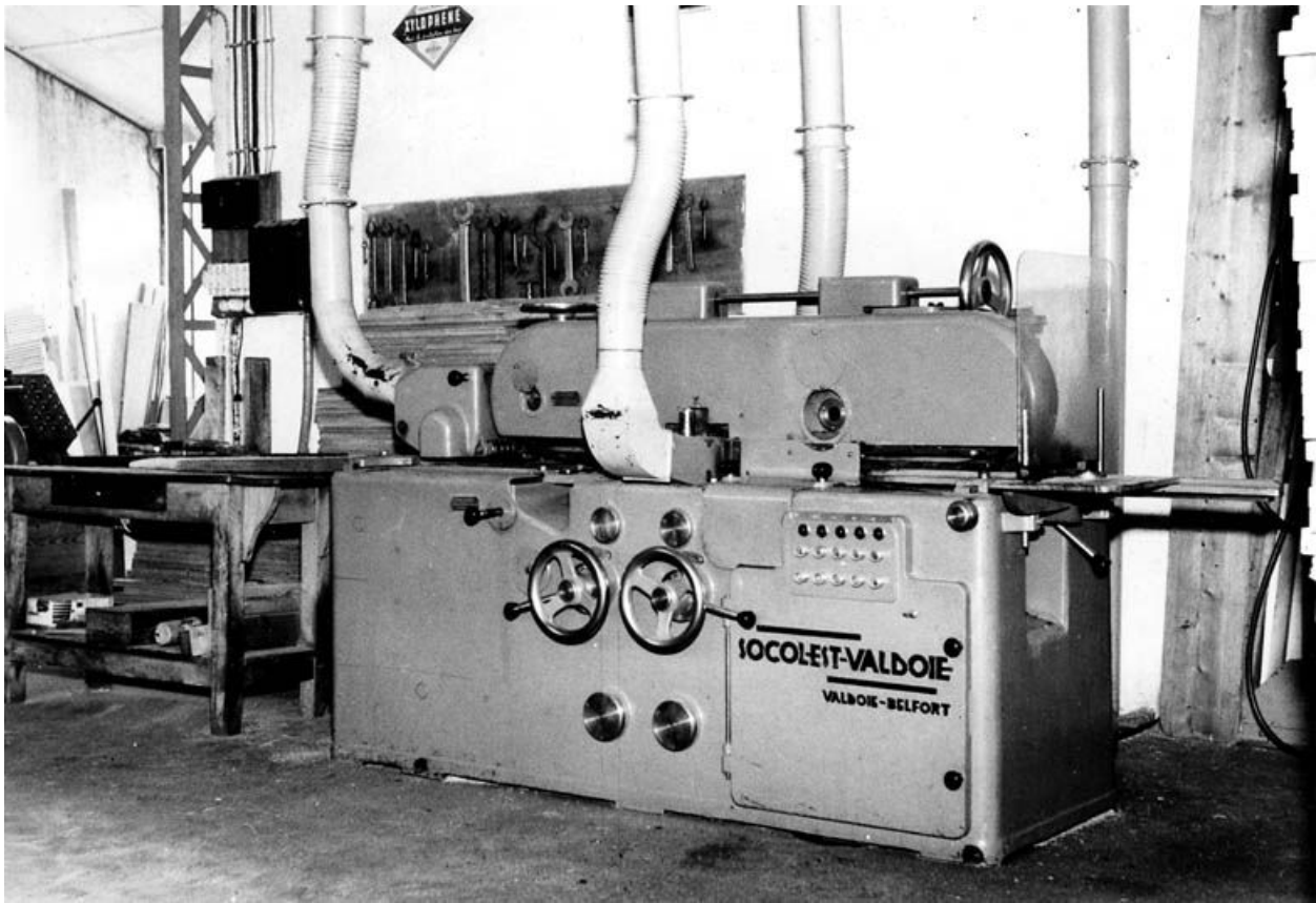
Vue intérieure de la parqueterie, machine à parquet 4 faces. Photographie. (Collection particulière)
