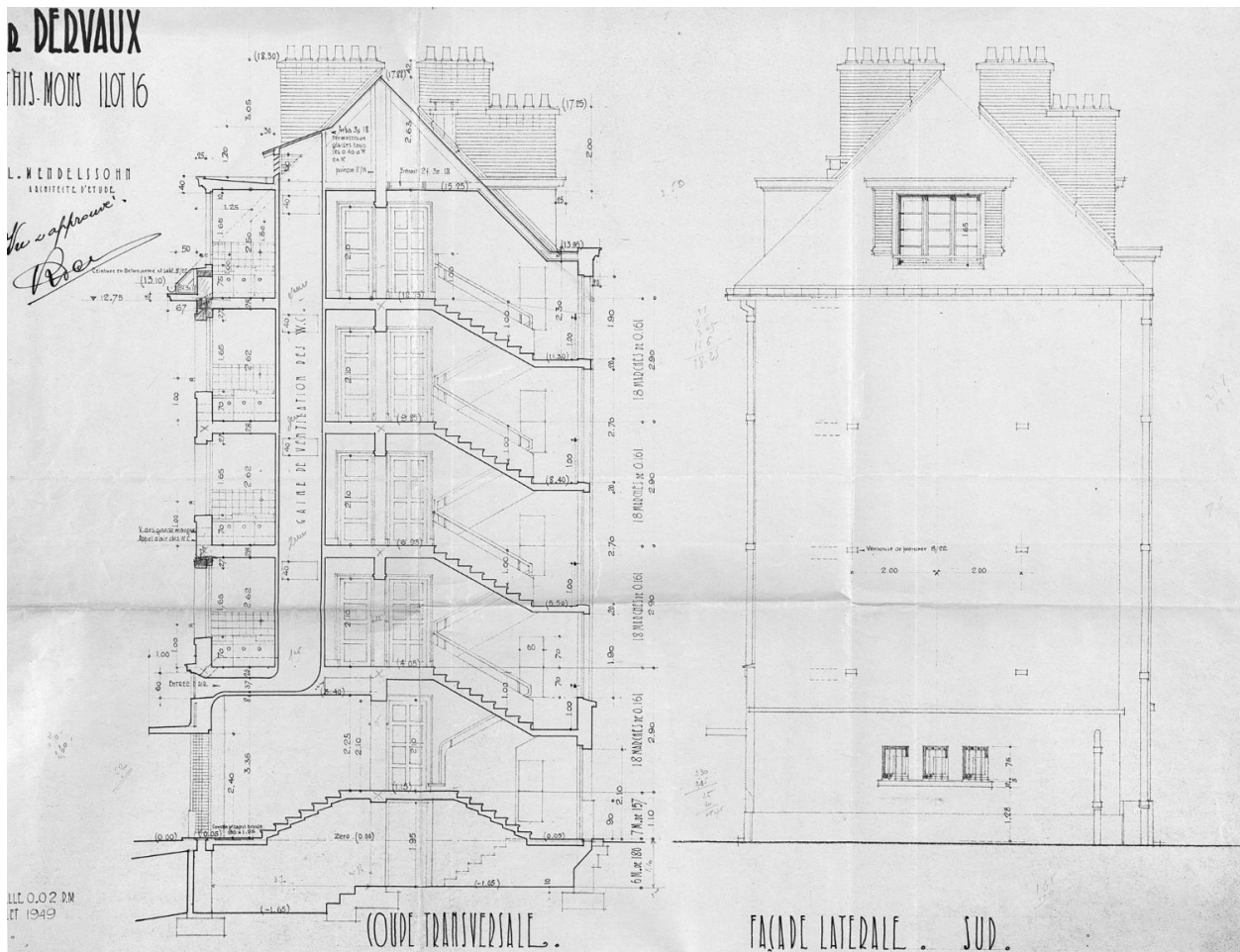
Coupe et élévation latérale de l'immeuble Dervaux (mitoyen de l'immeuble Clayeux), îlot 18/20bis, 2-4bis, place Jean-Jaurès ; Mendelssohn, architecte d'étude ; juillet 1949.
