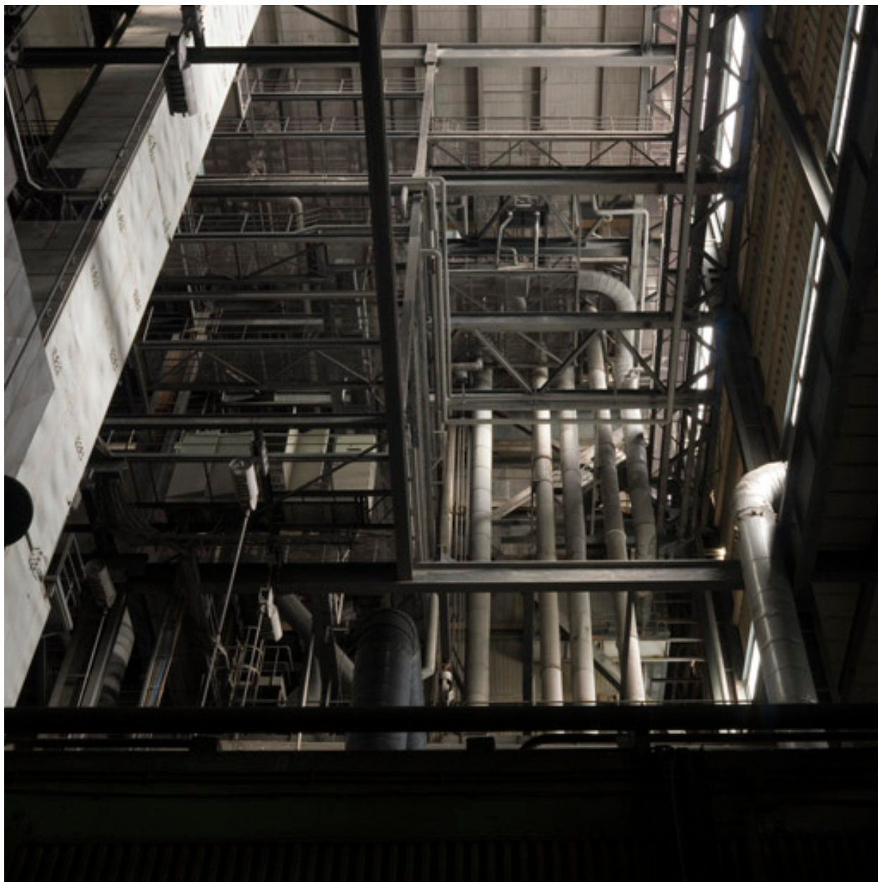
Générateur de vapeur 250 MW.
