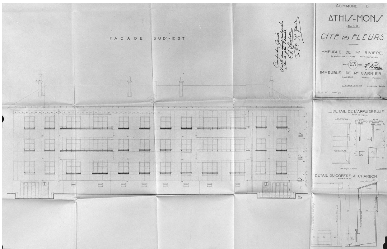
Plan de l'immeuble Rivière et Garnier, dressé par les architectes Mendelssohn, Blareau, Guillaume et Aubert, août 1953 : façade sud-est et détails de l'appui de baie et du coffre à charbon.
