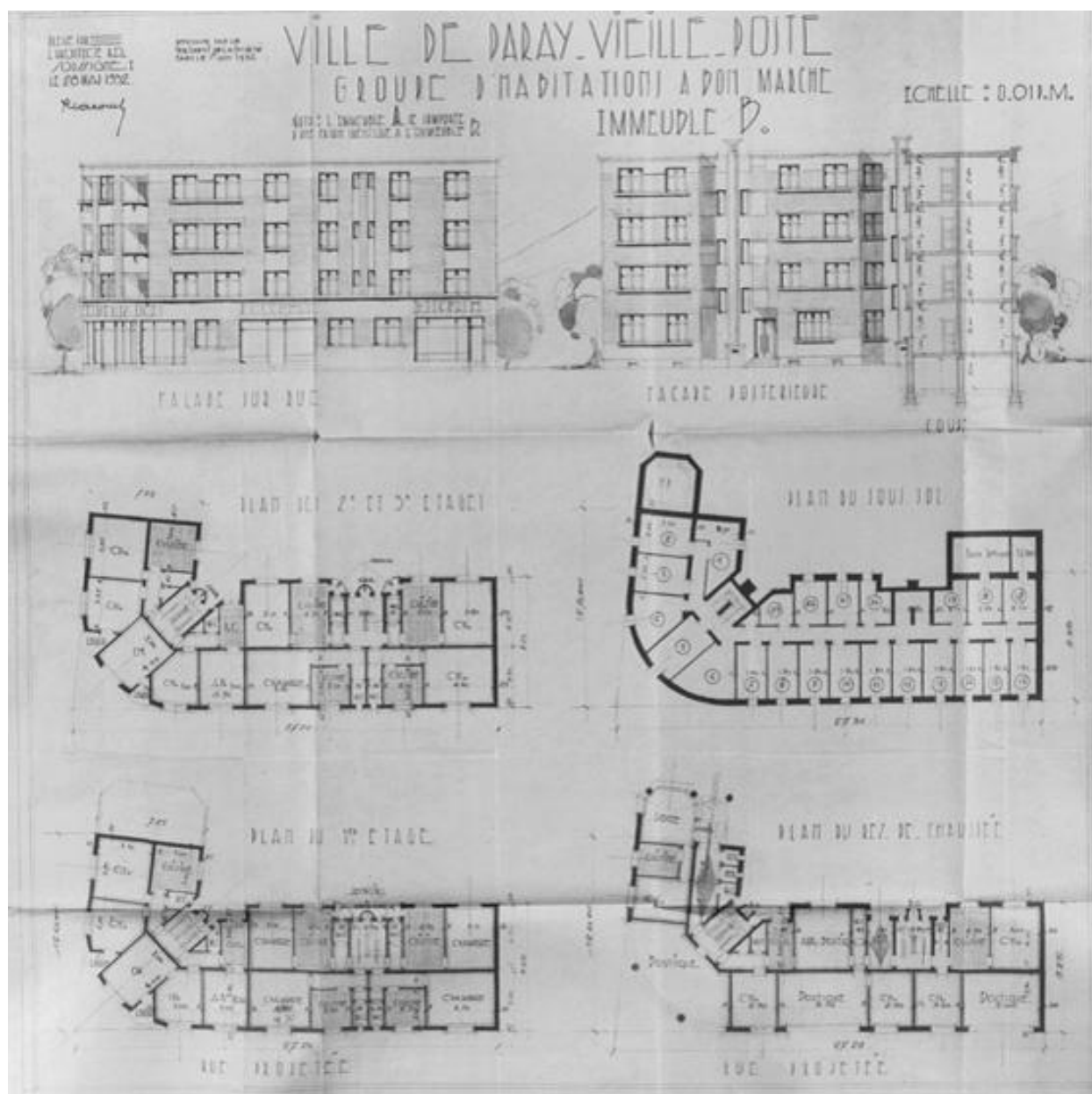
Immeubles A et B : élévations principale et postérieure, plans. 1er juin 1932.
