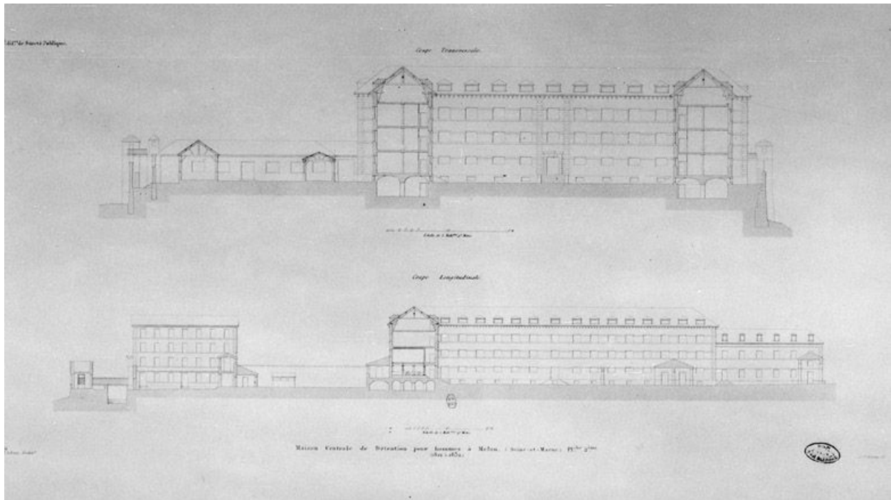
Coupes de la maison centrale, par l'architecte Solente, 1812 à 1832. (BNF, Département des estampes. Topo Va Seine-et-Marne)
