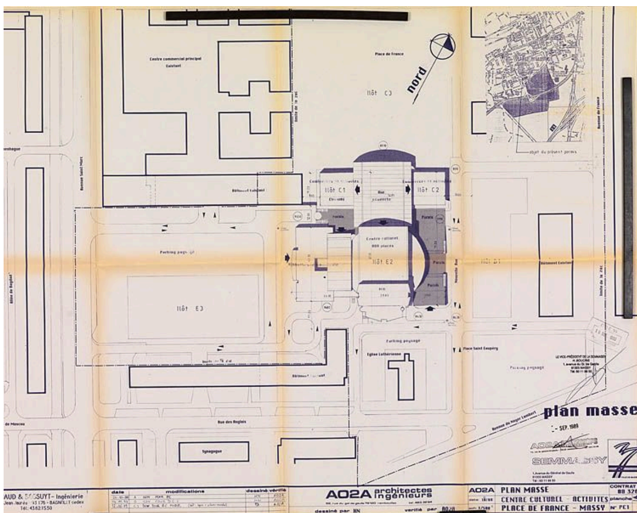
Plan masse de l'opéra. (AM Massy)
