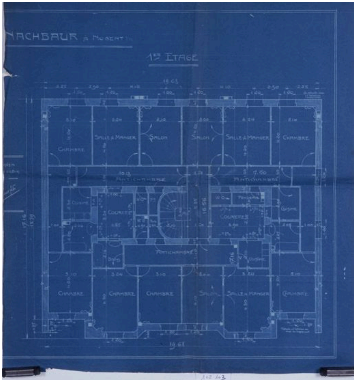
Plan de demande d'autorisation de construire pour Mr Nachbaur. Plan du 1er étage. Signé et daté Nachbaur mai 1912. (AM Nogent-sur-Marne. 1 02 103)
