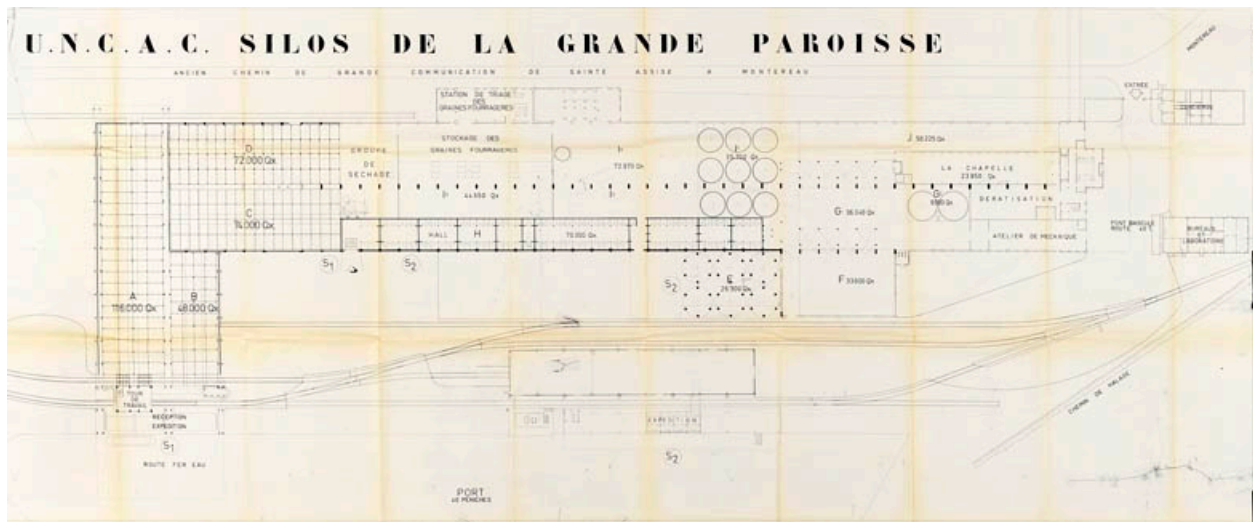
Silos de l'UNCAC de la Grande Paroisse. Plan masse. (Archives départementales).
