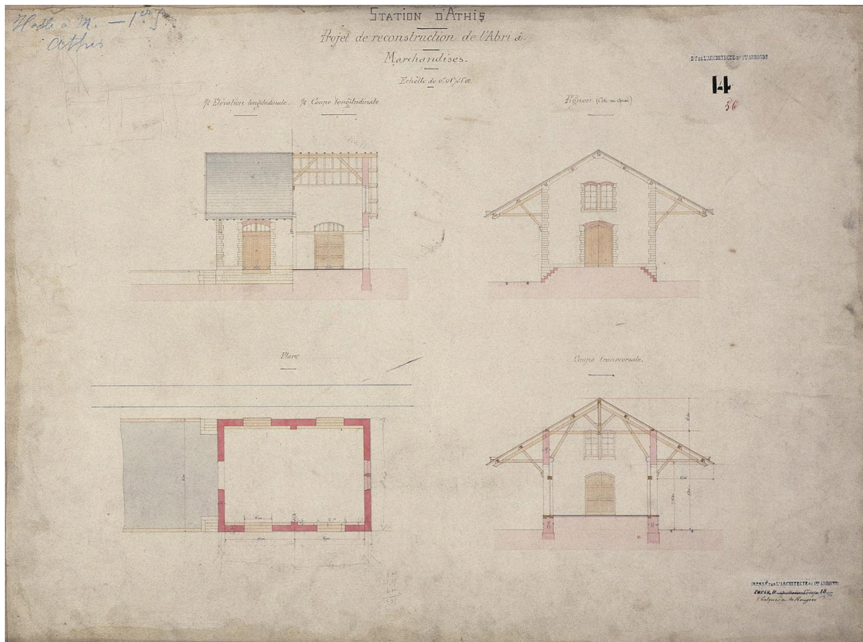
Projet de reconstruction de l'abri à marchandises : plan, coupes et élévations ; s.d. [vers 1870].
