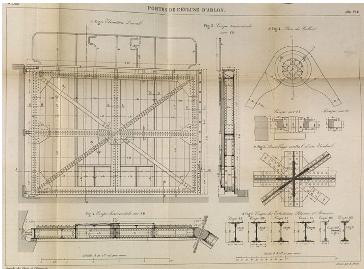
Ablon-sur-Seine, Vigneux-sur-Seine. Barrage éclusé d'Ablon-sur-Seine. Portes de l'écluse d'Ablon. Tiré de : Notice sur les portes de l'écluse d'Ablon / M. Lavollée. In Annales des Ponts et Chaussées, 1er semestre 1882, n° 30, pl. 6.
