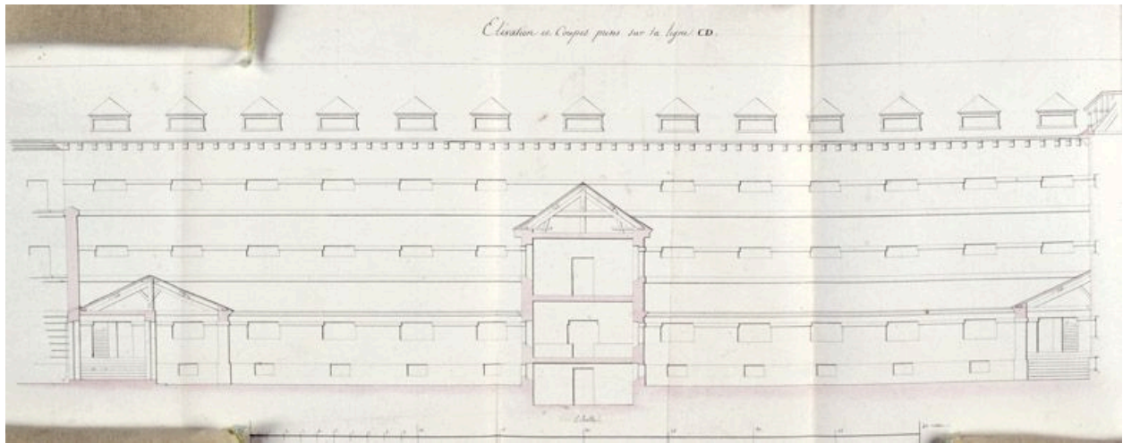
Elévation du grand bâtiment projeté par Solente, architecte départemental. Papier aquarellé, 1818. (AD Seine-et-Marne. 1 Y 52)
