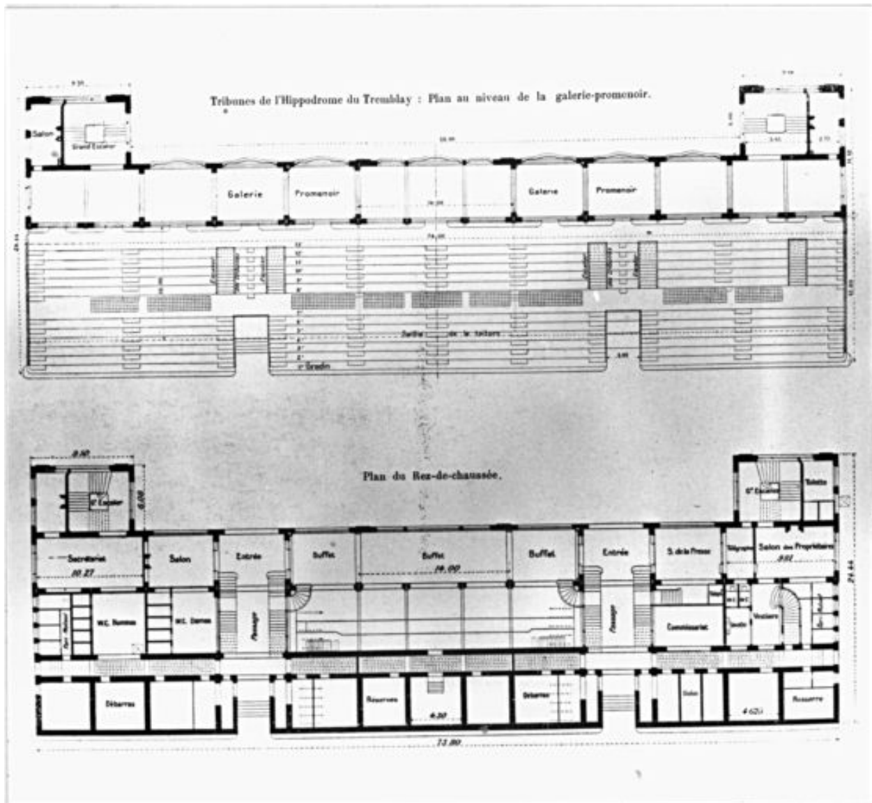
Plan du rez-de-chaussée (en bas) et du niveau de la galerie-promenoir des tribunes. Tiré de : La construction moderne, 1906-1907. (BNF. Estampes, topo Va 94, fol., t.3, B 14277)
