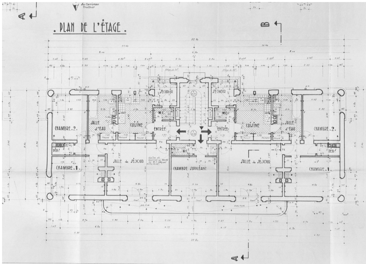
Logement des instituteurs : plan de l'étage ; Mendelssohn et Thivier et Poggi, architectes, mars 1951.
