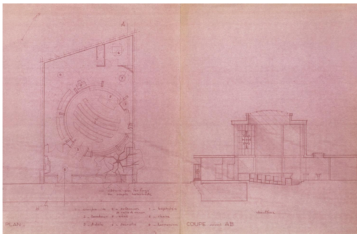
Projet de Claude Le Coeur en 1948 : plan d'ensemble et coupe, 3 mai 1948.
