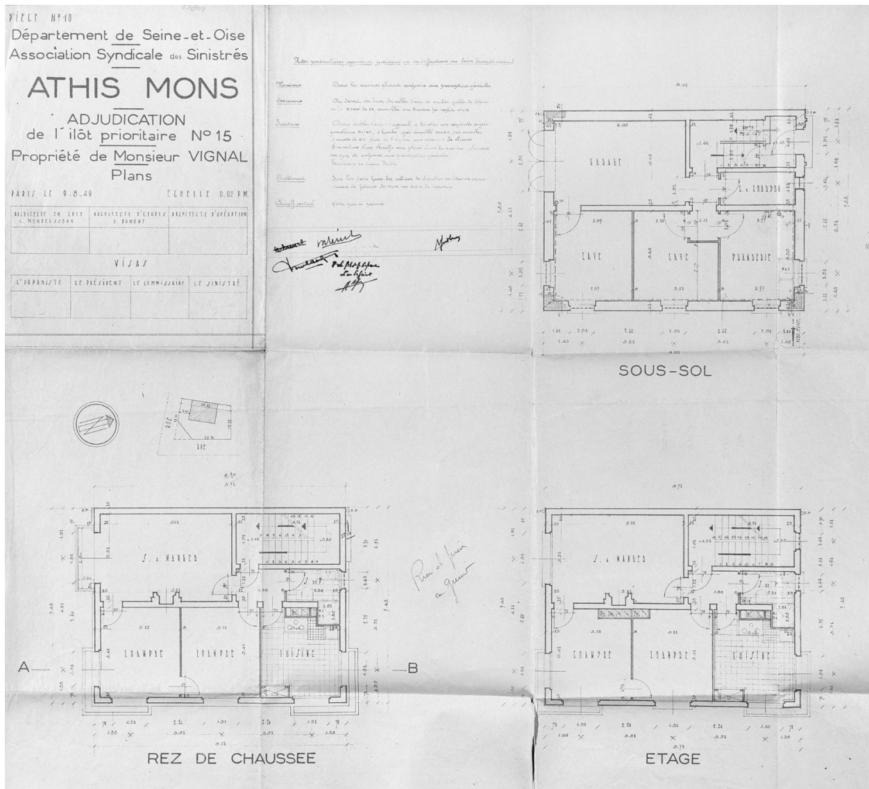
Plans (sous-sol, rez-de-chaussée et étage) de la maison reconstruite dans l'îlot 15 pour M. Vignal (59, avenue Jean-Jaurès) ; architecte en chef Léo Mendelssohn, G. Dumont, architecte d'études, Chavany, architecte d'opération, 9 août 1949.
