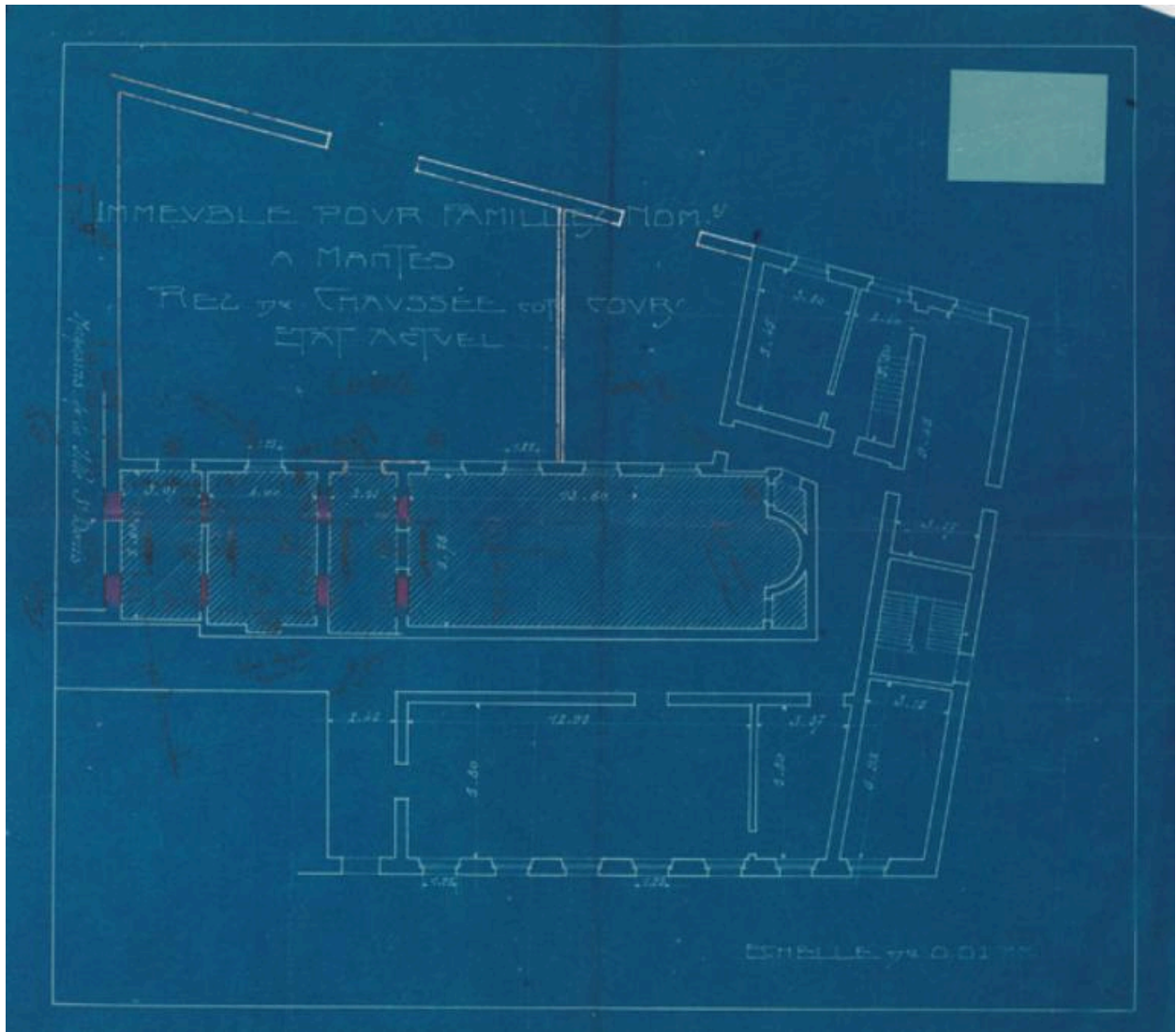
Plan du RDC côté cour de l'immeuble pour familles nombreuses, Cauzard, Marabout (architectes), non daté (1922 ?), (AM Mantes-la-Jolie, 7M 2(2)).
