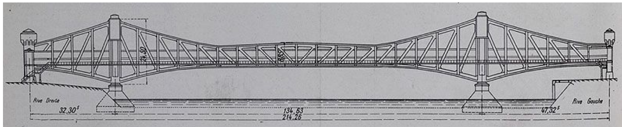
Ivry-sur-Seine, Charenton-le-Pont. Passerelle industrielle d'Ivry-Charenton. Elévation schématique cotée. Tiré de : Travaux, juillet 1939, p. 280.
