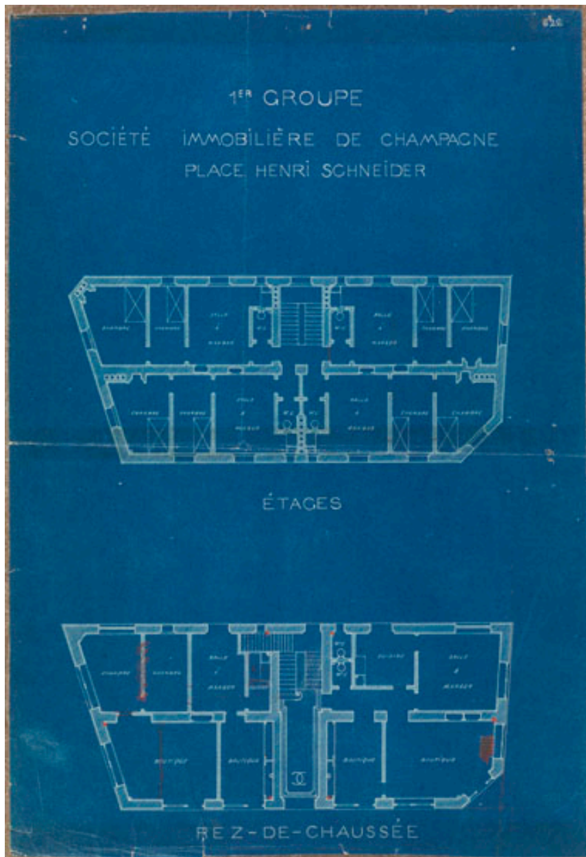
Plan. Société immobilière de Champagne. Etage et rez-de-chaussée. 1er groupe, place Henri Schneider.
