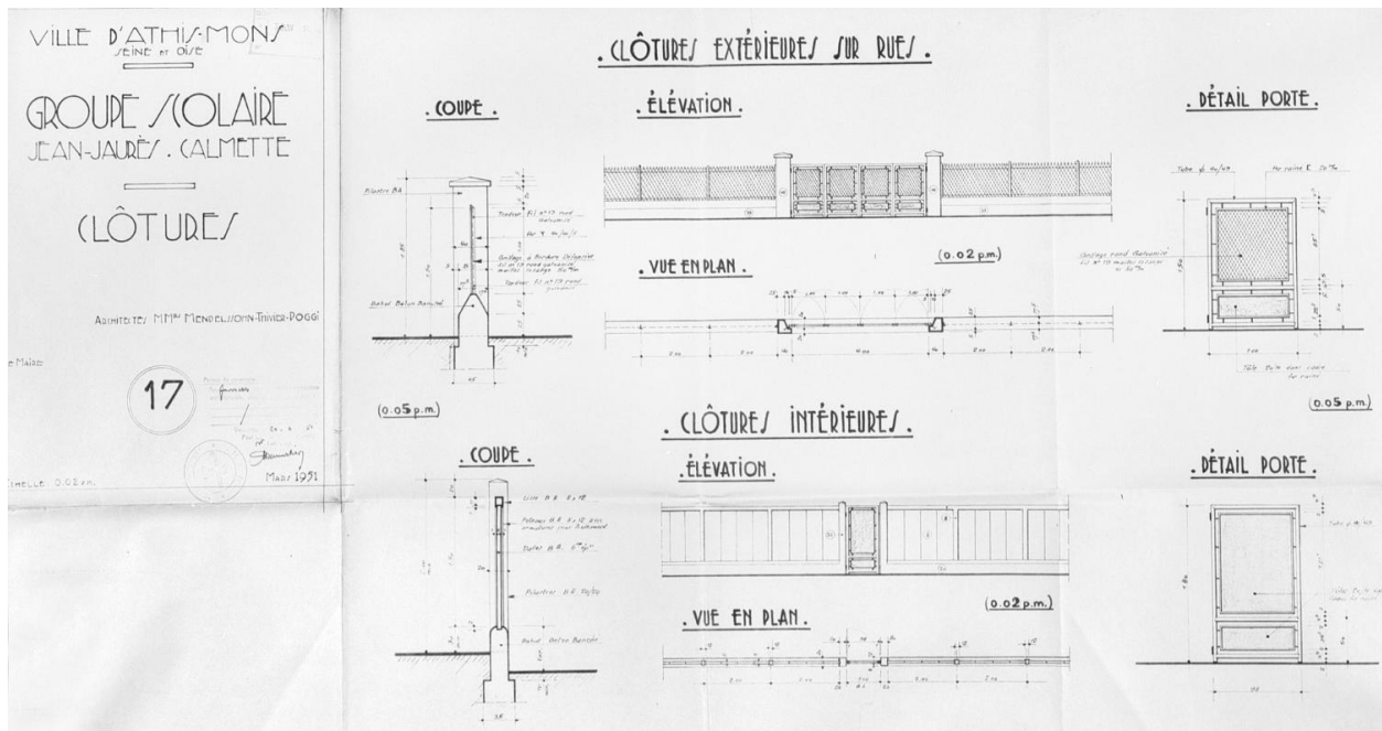
Clôtures intérieures et clôtures extérieures sur rue : élévations, coupes, vues en plan et détail des portes ; L. Mendelssohn, Thivier et Poggi architectes, mars 1951.
