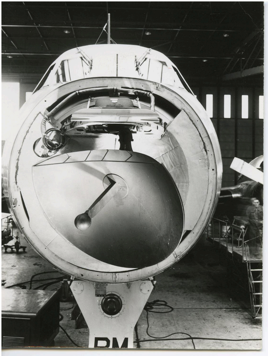
Vers 1960, zone industrielle nord de l'aéroport d'Orly, opération de maintenance sur le radar d'un Boeing 707 d'Air France.
