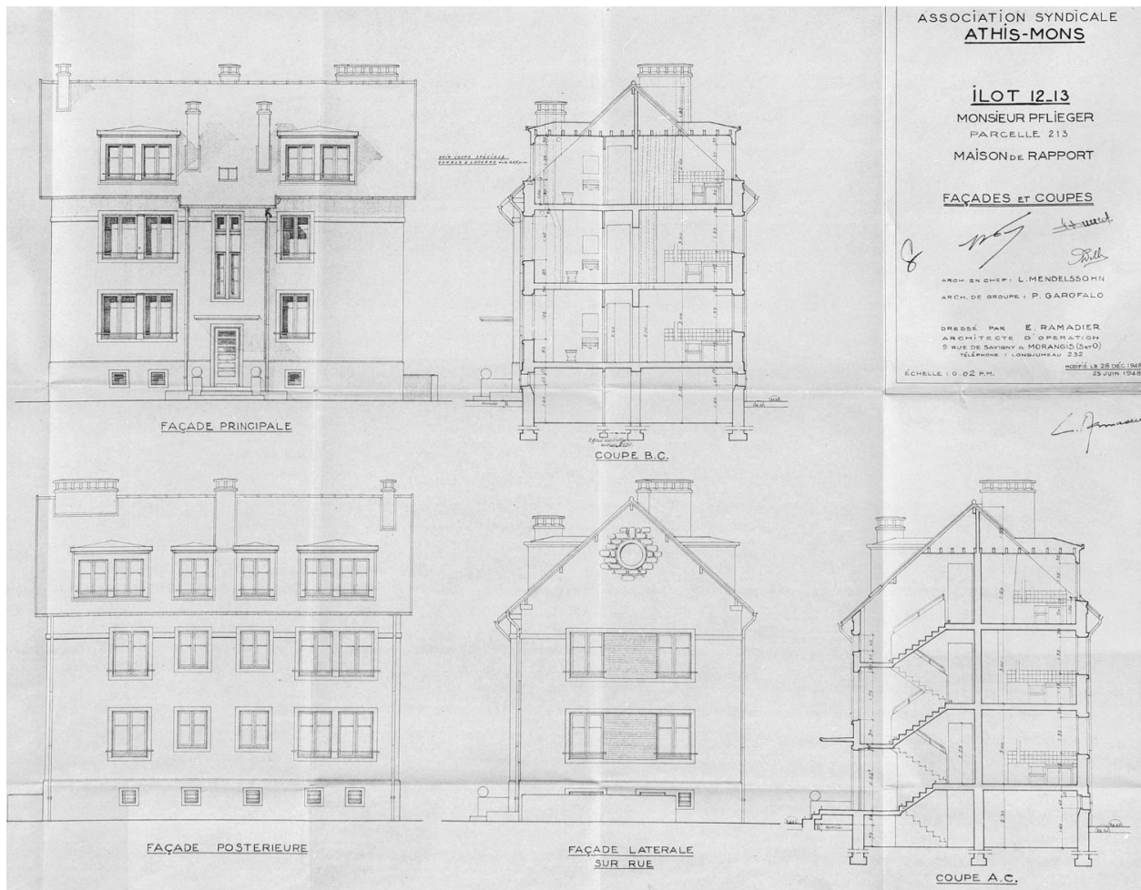
Elévations et coupe de l'immeuble reconstruit pour M. Pflieger dans l'îlot 12-13, parcelle 213, par E. Ramadier, architecte d'opération, 25 juin 1948.
