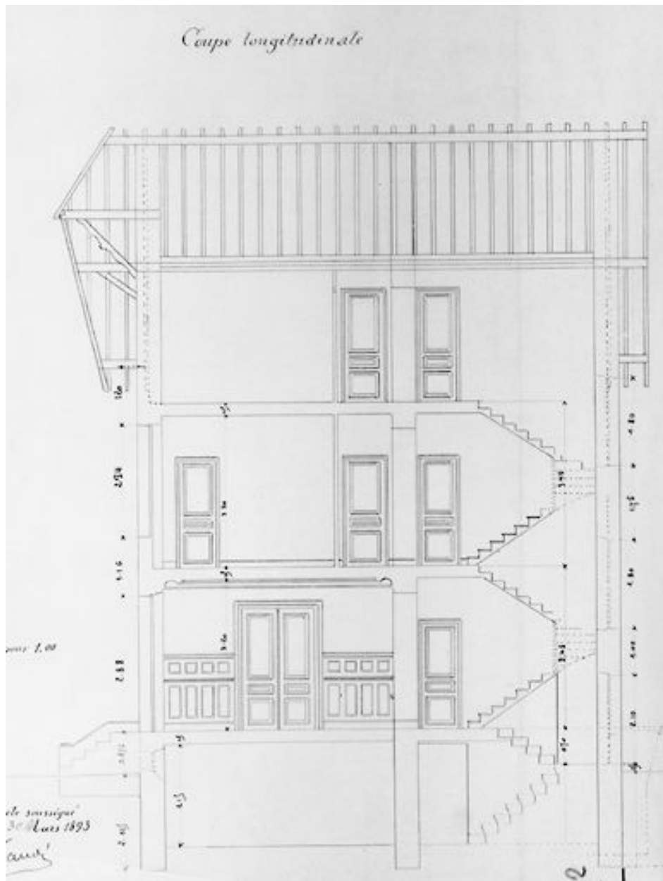
Projet pour la propriété de M. Matras, rue de Dammarie : coupe longitudinale. Encre sur calque, 30 mars 1893. (AM Melun. 1 Fi 825)
