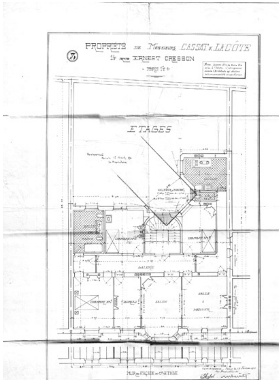
Etages, propriété de Messieurs Cassat et Lacôte. -Plan, 1911. (Archives de Paris, VO11 1131).
