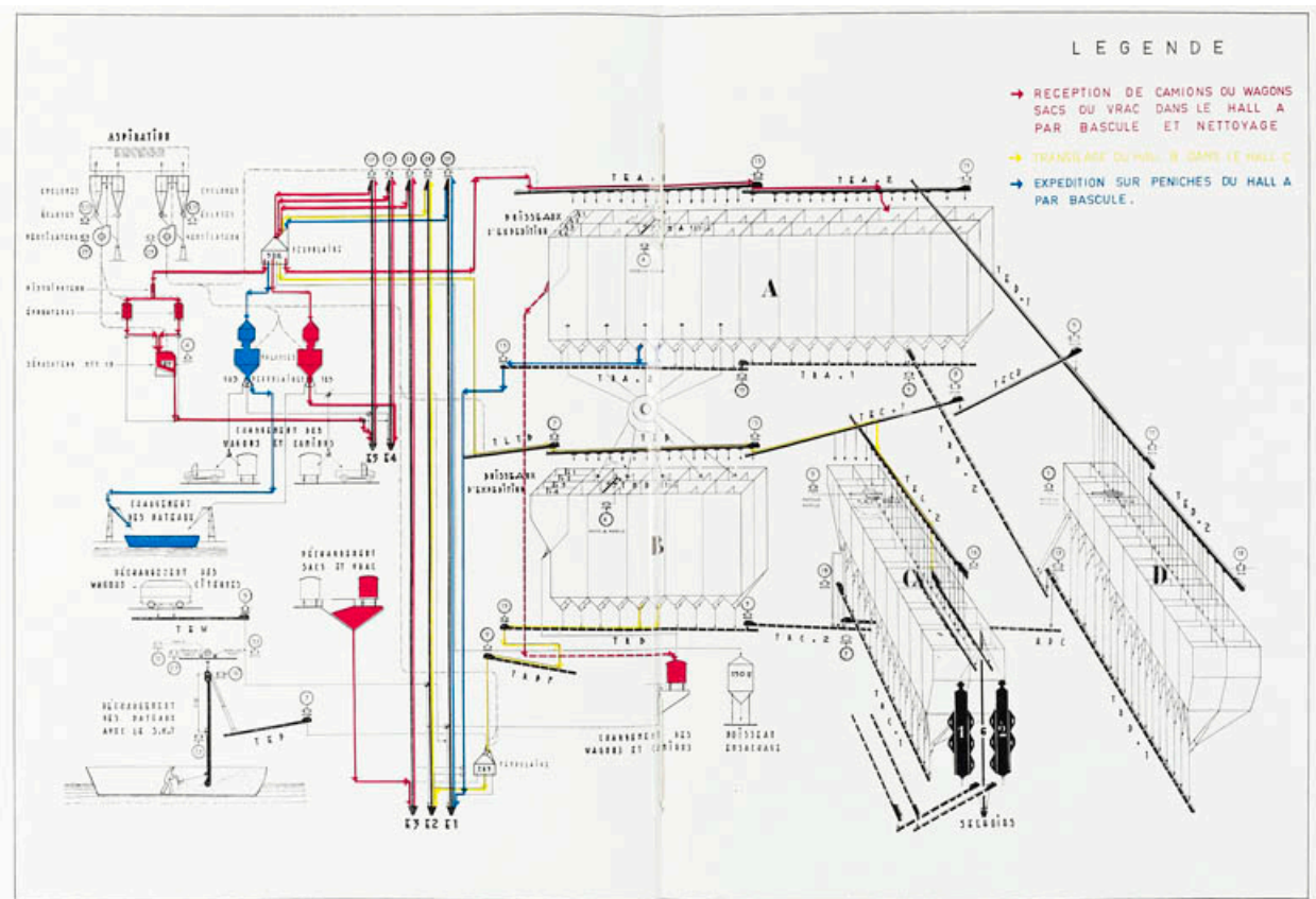
Schéma de l'organisation du silo. (Archives départementales).
