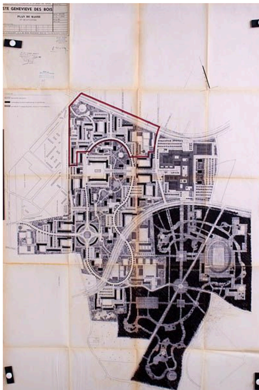
Cité dite Résidence Saint-Hubert. Plan masse de la résidence Saint-Hubert.
