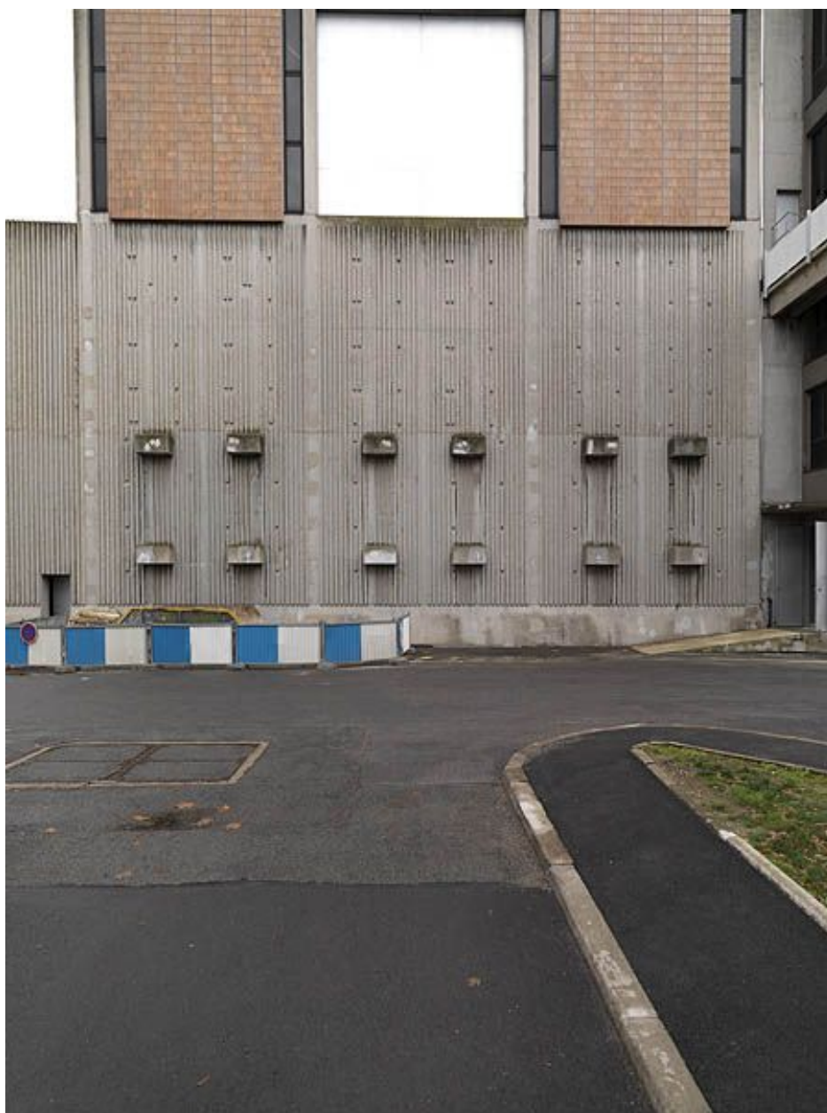
Choisy-le-Roi, établissement des eaux dit usine de traitement des eaux de Choisy. Détail de mise en oeuvre du béton.
