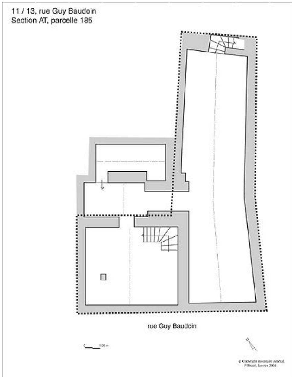
Plan de la cave du 11-13 rue Guy-Baudouin.
