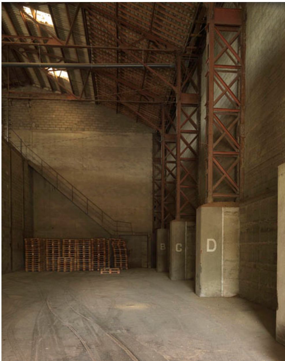
Silos de l'UNCAC de la Grande Paroisse, aujourd'hui Invivo. Vue intérieure du Silo 2, ancienne centrale électrique de la cimenterie Polliet et Chausson.
