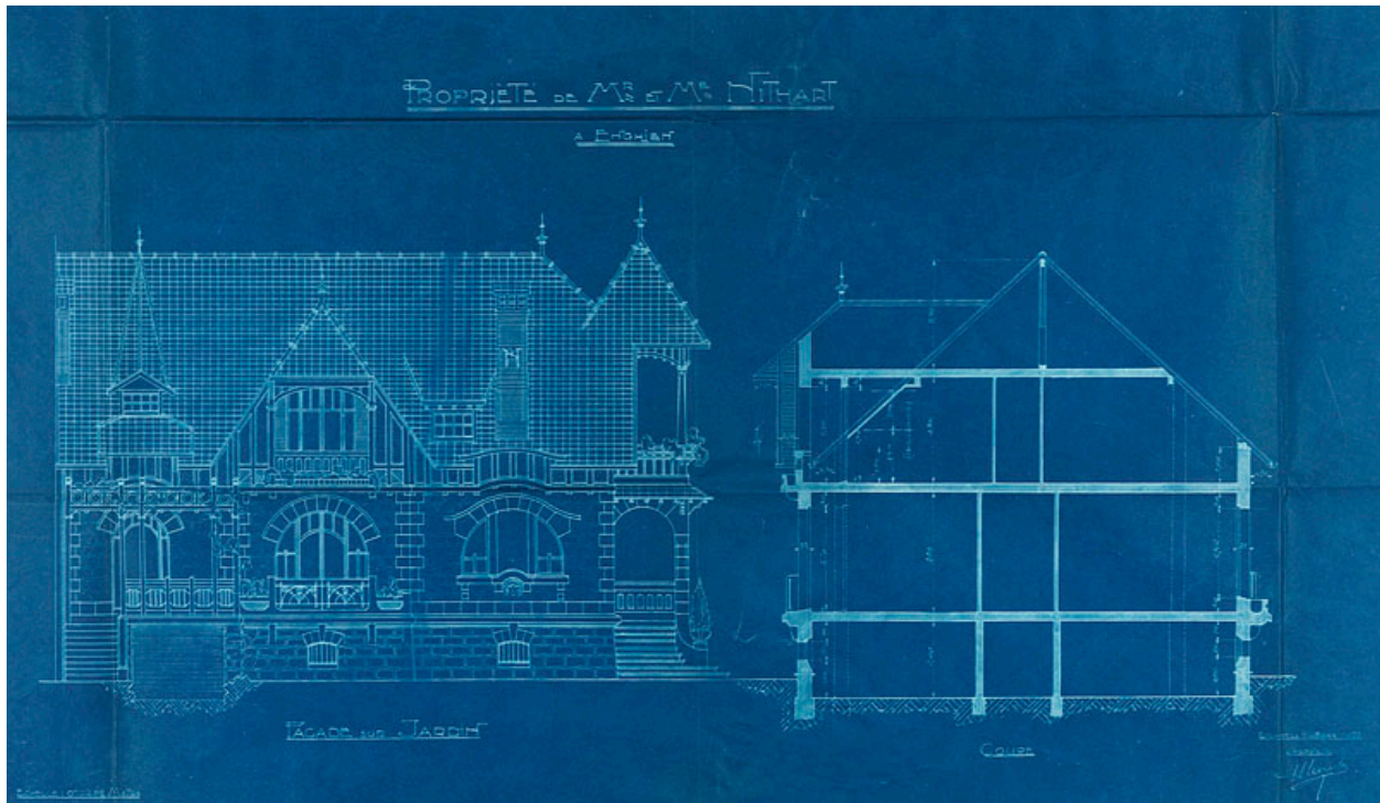
Élévation de la façade sur jardin et coupe, 1925. (AM Enghien-les-Bains, 1T 134)
